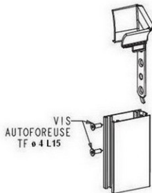
fixation par vis
